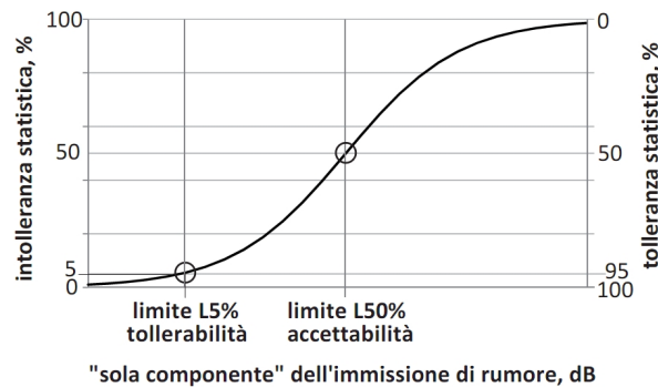
Figura 6 – L'intolleranza 5% è raggiunta con rumore al limite della tollerabilità L 5% . L'intolleranza 50% con rumore al limite dell' accettabilità L 50% .
