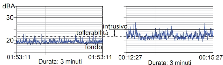
Figura 1 - I picchi della musica del pub e il limite della tollerabilità dei 3 dB.
